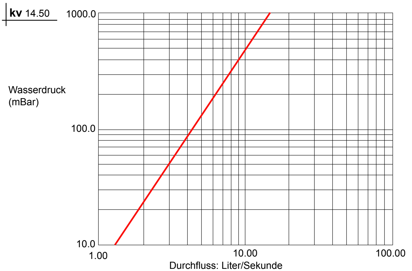
Diagramm 990844/TA/3: Angabe vom Druckverlust durch den magnetischen Entkalker ELCLA5 Ø 2".
