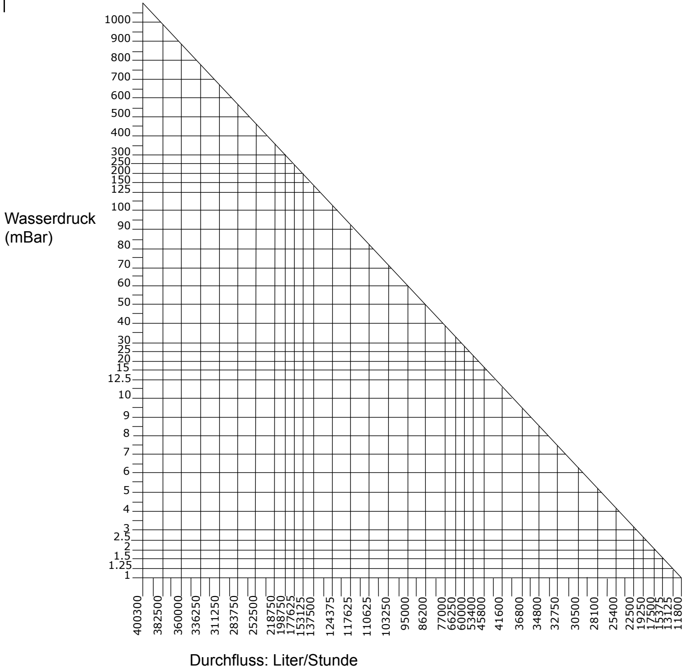
Diagramm TEST 0403102/GS/3: Angabe vom Druckverlust durch den magnetischen Entkalker ELCLA8 DN 100 Ø 4".
