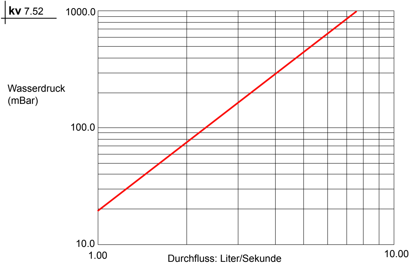
Diagramm 990844/TA/1: Angabe vom Druckverlust durch den magnetischen Entkalker ELCLA4 Ø 1.1/4".
