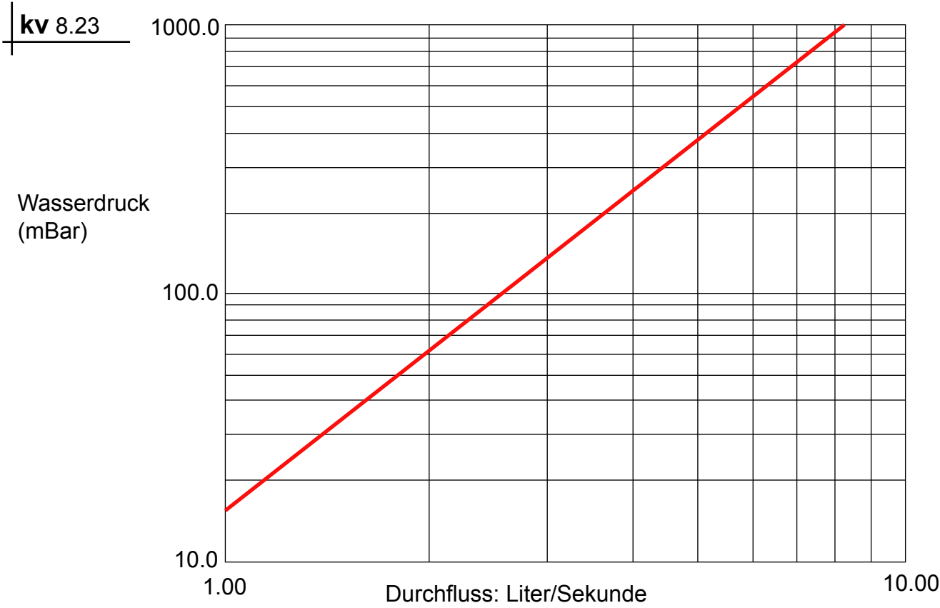
Diagramm 990844/TA/2: Angabe vom Druckverlust durch den magnetischen Entkalker ELCLA4A Ø 1.1/2".
