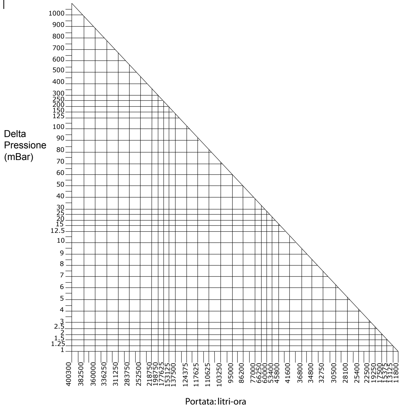
Diagramma TEST 0403102/GS/3: determinazione della perdita di carico contro portata dell'anticalcare magnetico ELCLA8 DN 100 Ø 4".
