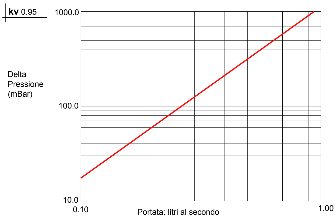
Diagramma 981559/1: determinazione della perdita di carico contro portata dell'anticalcare magnetico MiniElcla Ø 1/2" e 3/4".
