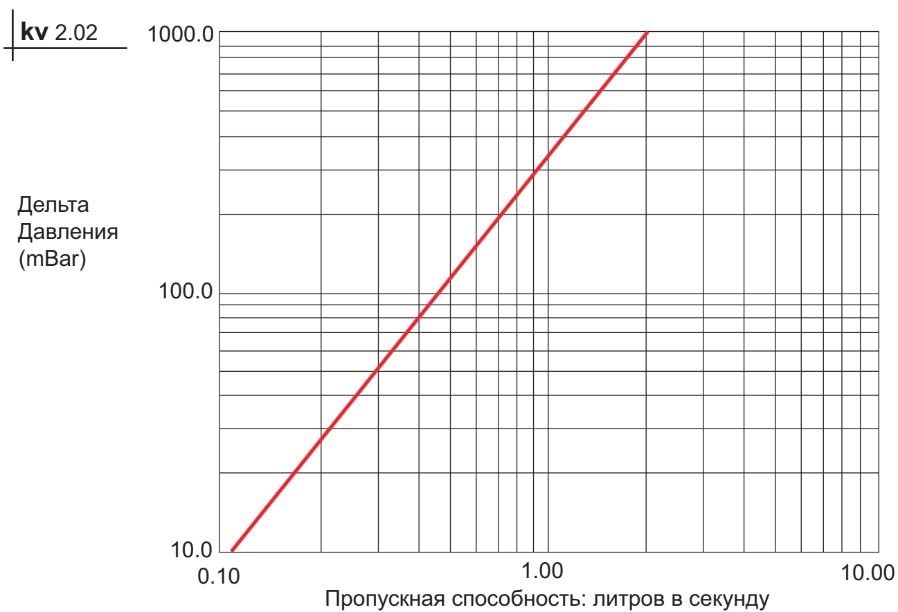
Диаграмма 981559/2: зависимость падения загрузки от пропускной способности магнитного противоиловного аппарата ELCLA1 Ø 1/2".
