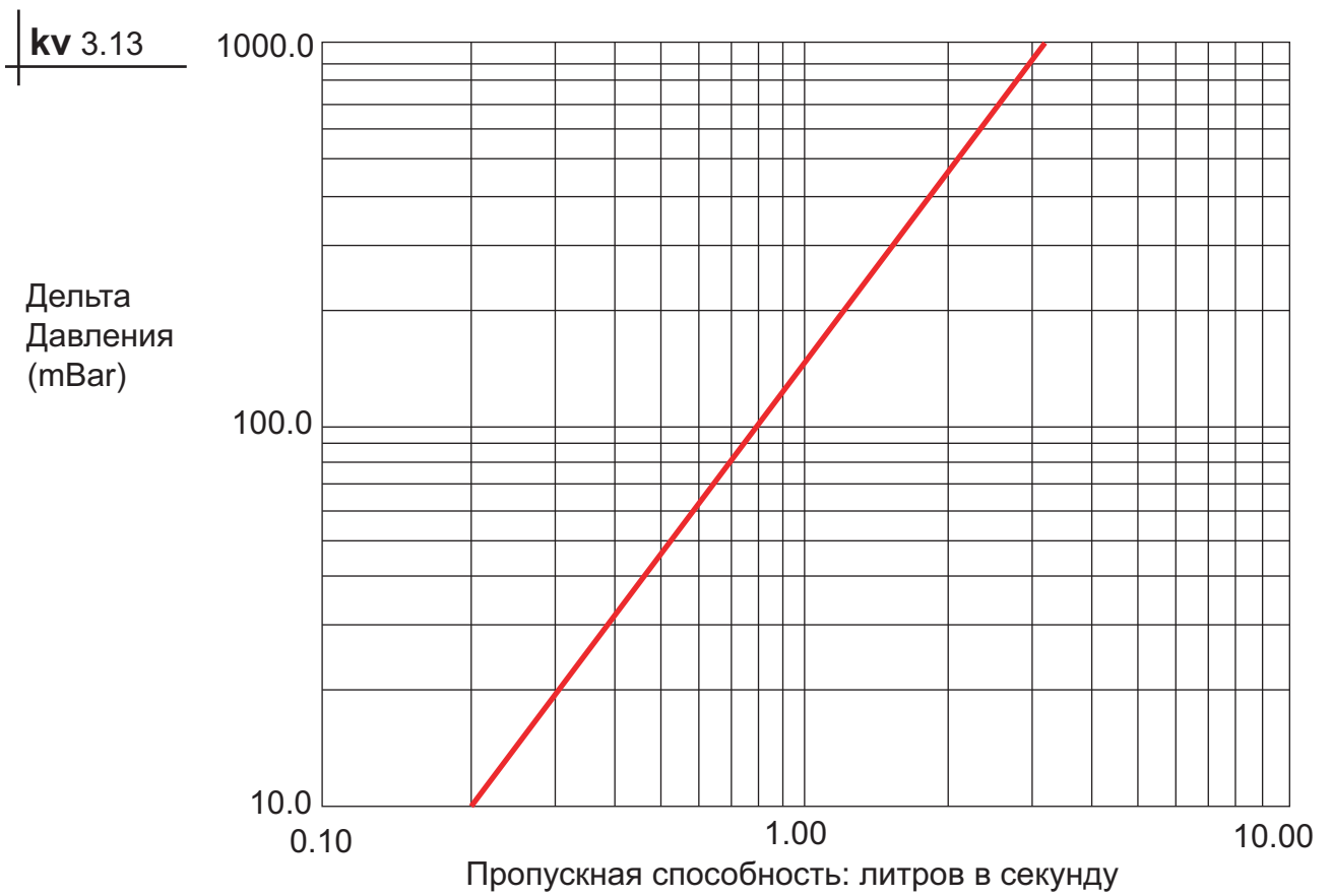
Диаграмма 981559/4: зависимость падения загрузки от пропускной способности магнитного противоиловного аппарата ELCLA3 Ø 1".
